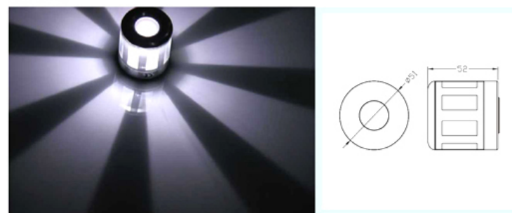
MS-WL51A
